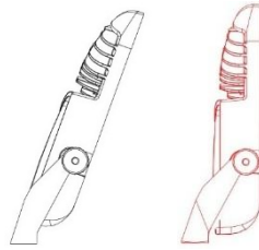
نصب عمودی
